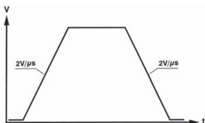
Anstiegs- und Abfallgeschwindigkeit bei TOE 8815 bis TOE 88165
