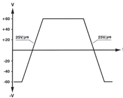
Anstiegs-/Abfallgeschwindigkeit bei TOE 7610-60
