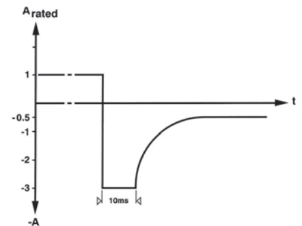
Kurzlast-Senke Option TOE 8810/107
