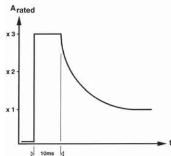
Kurzlaststrom mit Option TOE 8810/103
