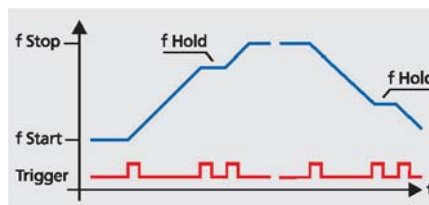
Getriggertes Sweep mit getriggertem Hold und getriggertem Reverse
