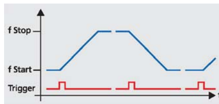
Getriggertes Sweep mit Hold und getriggertem Reverse
