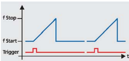
Getriggertes Sweep mit Reset
