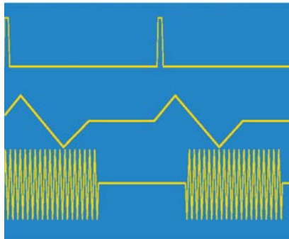
Ausgangssignale bei Trigger- und Gatebetrieb
