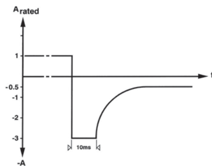
Kurzlast-Senke Option TOE 8810/107
