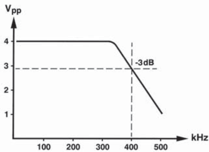
Kleinsignalbandbreite bei TOE 7610
