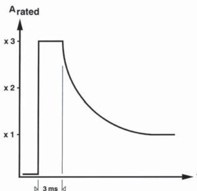
Kurzlaststrom 3 \times I_{Nenn} bei TOE 7610 (Option TOE 7610/103)
