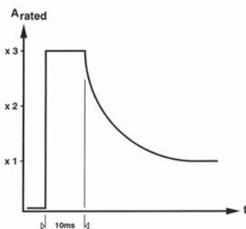
Kurzlaststrom 3 \times I_{Nenn} Option TOE 8810/103
