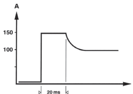
Kurzlaststrom bei TOE 8872-40 (Option TOE 8871/022)
