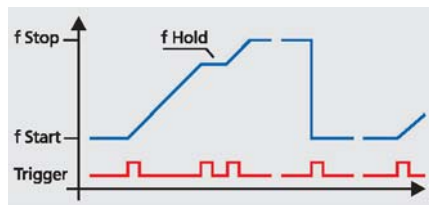
Getriggertes Sweep mit getriggertem Hold und getriggertem Reset
