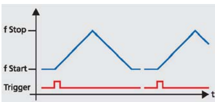
Getriggertes Sweep mit Reverse
